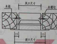
外木框安装法 (一)
