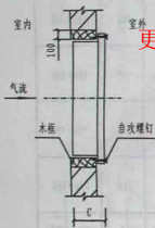
壁式风机安装 A
