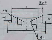
YS (圆环型)
