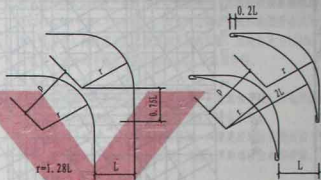
单层做法
