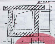
混凝土预制框立面图
