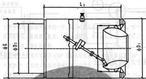
内置执行器球形可调喷口
