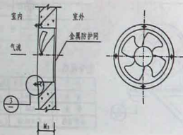
墙上安装
