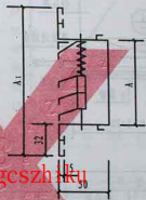
TF (活芯式)
