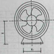
GYF-I 型
