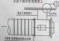
直接与圆形管道或软管对接
