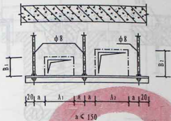
平行矩形不保温风管三杆吊架
