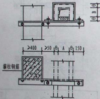
矩形保温风管柱上支架 (一)
