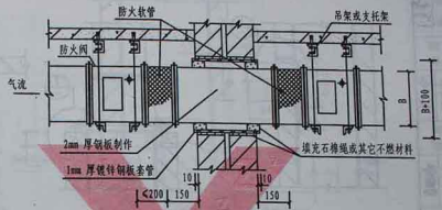
水平风管穿沉降缝做法
