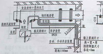
排烟口安装示意图
