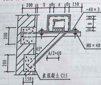
圆形不保温风管墙上支架
