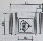
圆形机械式定风量阀 (非法兰口)
