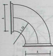
内外弧形矩形弯管
