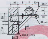
圆形保温风管墙上斜撑支架
