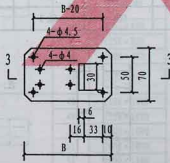
垫板
