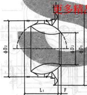
球形可调喷口
