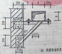
矩形不保温风管墙上斜撑支架
