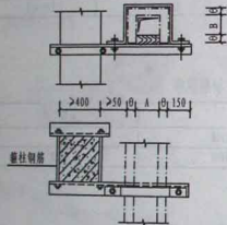
矩形保温风管柱上支架 (二)
