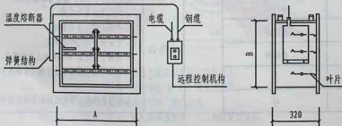
远控防烟防火调节阀 HAFH-17 型
