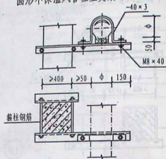
圆形保温风管柱上支架 (二)
