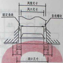
风管插入安装法
