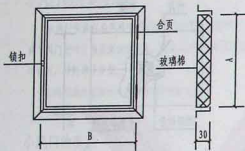
铝合金吊顶检查门
