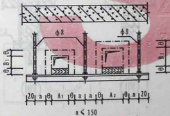
平行矩形保温风管三杆吊架
