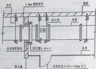
风管水平穿越防火分区分隔墙时防火阀的安装
