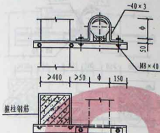
圆形不保温风管柱上支架 (一)
