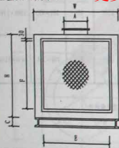
垂直出风外形图:
