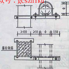
圆形保温风管柱上支架 (二)
