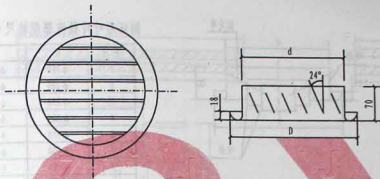
YS (斜片型)
