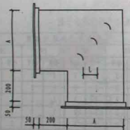
直角矩形弯管
