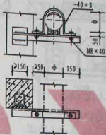
圆形不保温风管柱上支架 (三)
