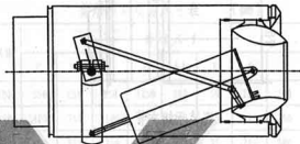
外置执行器球形可调喷口
