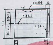
阀叶立面
