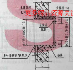
多叶排烟口/送风口在竖井壁上安装
