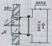
板式排烟口在墙上与铁皮风道安装
