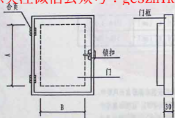
管道修理门
