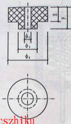
橡胶减振器
