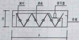
双层叶片钢制人字风阀
