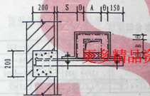
矩形不保温风管墙上斜撑支架
