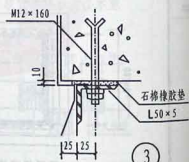
C. 土建风道下接风管
