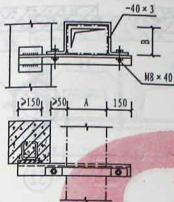
矩形不保温风管柱上支架 (三)
