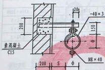
圆形不保温风管墙上吊架
