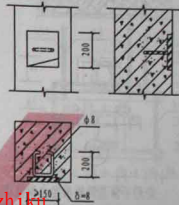
柱中预埋件大样
