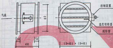
圆形防火调节阀
