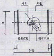
圆形风管小风门
