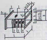
1. 外部保护壳 2. 保温材料 3. 法兰 4. 骨架 5. 防火防霉软管材料
