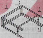
自撑式风管龙骨架
