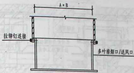
多叶排烟口/送风口与钢板风管连接
