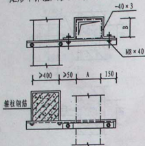
矩形不保温风管柱上支架 (一)
