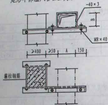
矩形保温风管柱上支架 (二)
