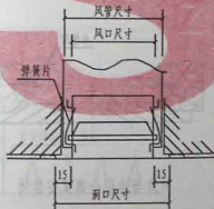
弹簧片安装法
