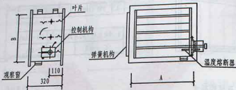
防火阀 HAFH-1 型
