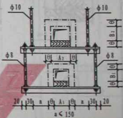
上下矩形保温风管吊架
