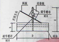
单向圆形风阀
