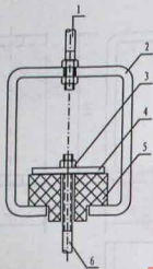
XTG 型弹性吊架
