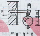
圆形保温风管墙上吊架
