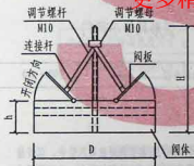
双向圆形风阀
