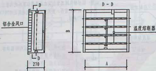
防火风口 HAFH-15 型
