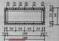
3h铁皮风管包覆截面图
