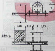
圆形保温风管柱上支架 (一)
